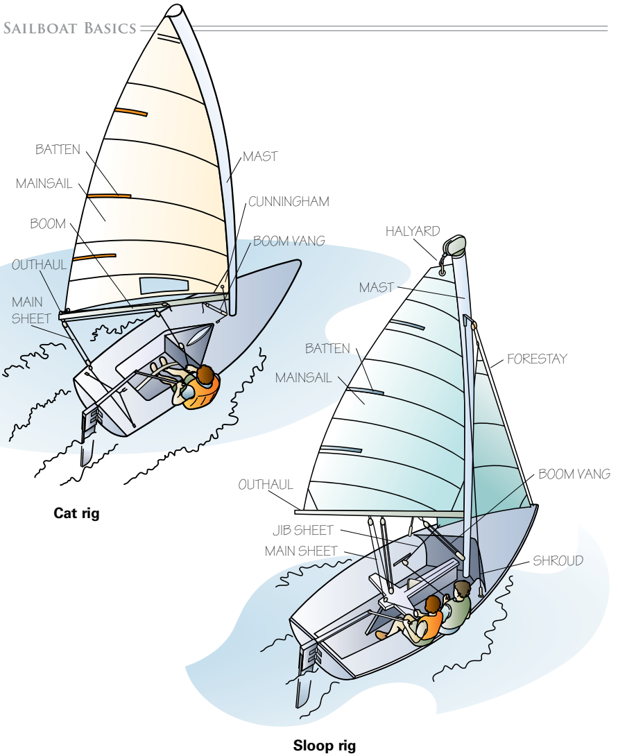
Sloop rig
